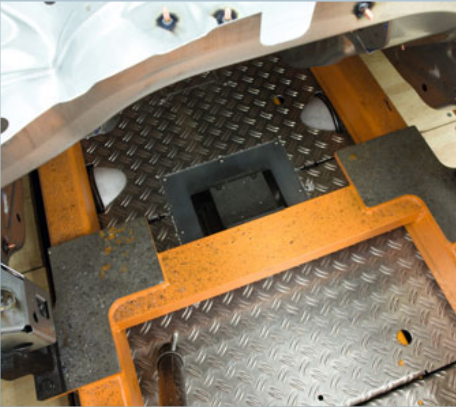
Das Identifikationssystem Simatic RF300 von Siemens sorgt dafür, dass die richtigen Komponenten zur richtigen Karosserie verbaut werden
